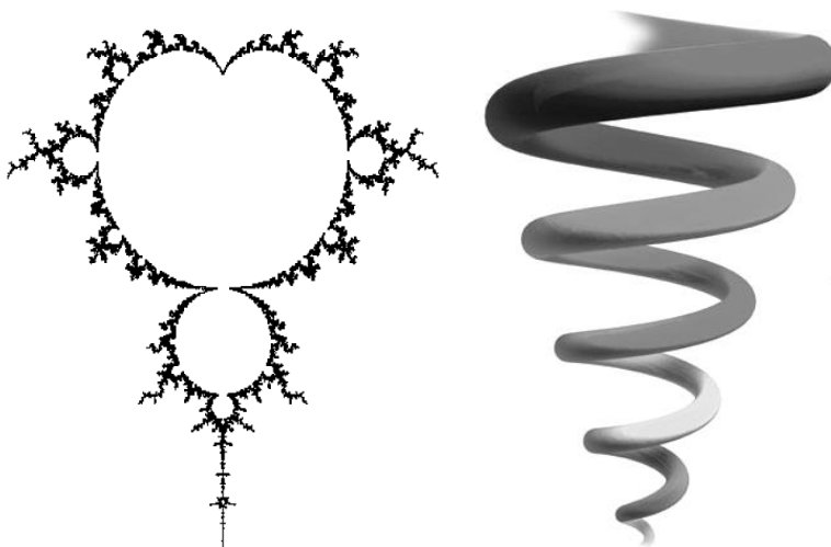
Рис. 3. Фрактал и затухающая спираль.
