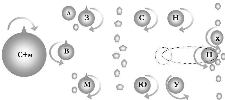
Рис. 76. Схема взаимодействия вращений планет после разрушения системы Фаэтон/Люцифер.
