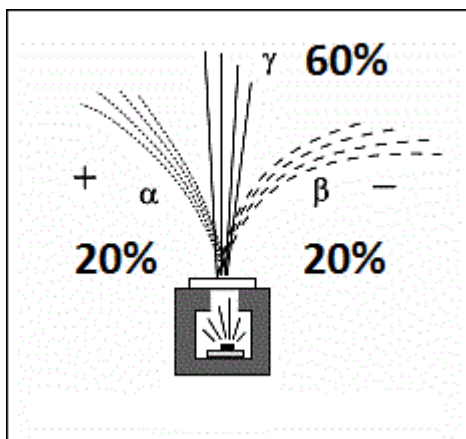
Рис. 19. Условия системной гармонии.
