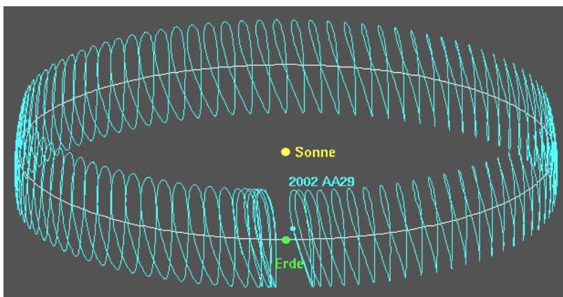
Рис. 7. Схема орбиты полета объекта 2002 AA29 вокруг Земли на ее орбите вокруг Солнца.
