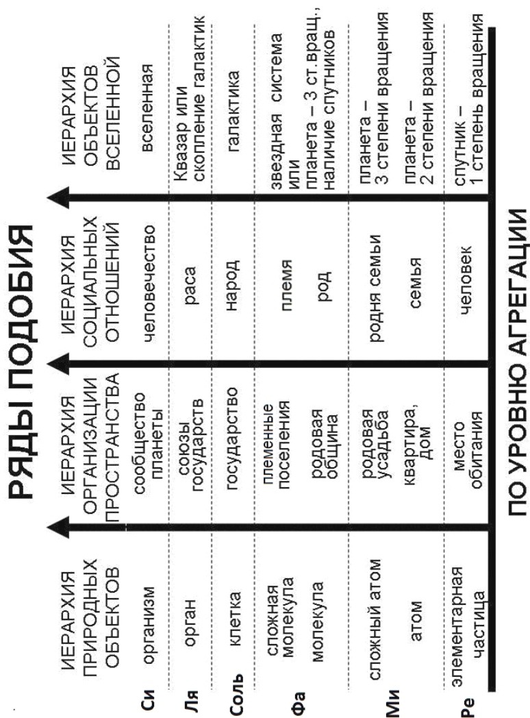
Рис. 9. Ряды подобия, построенные по уровню агрегации материи и социальных систем во вселенной.
