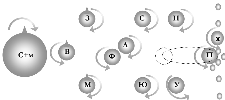
Рис. 7а. Схема взаимодействия вращений планет до разрушения системы Фаэтон/Люцифер.
